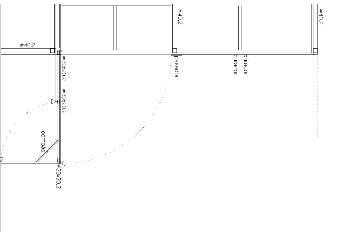
SECCIÓN ZONA APERTURA MESA
